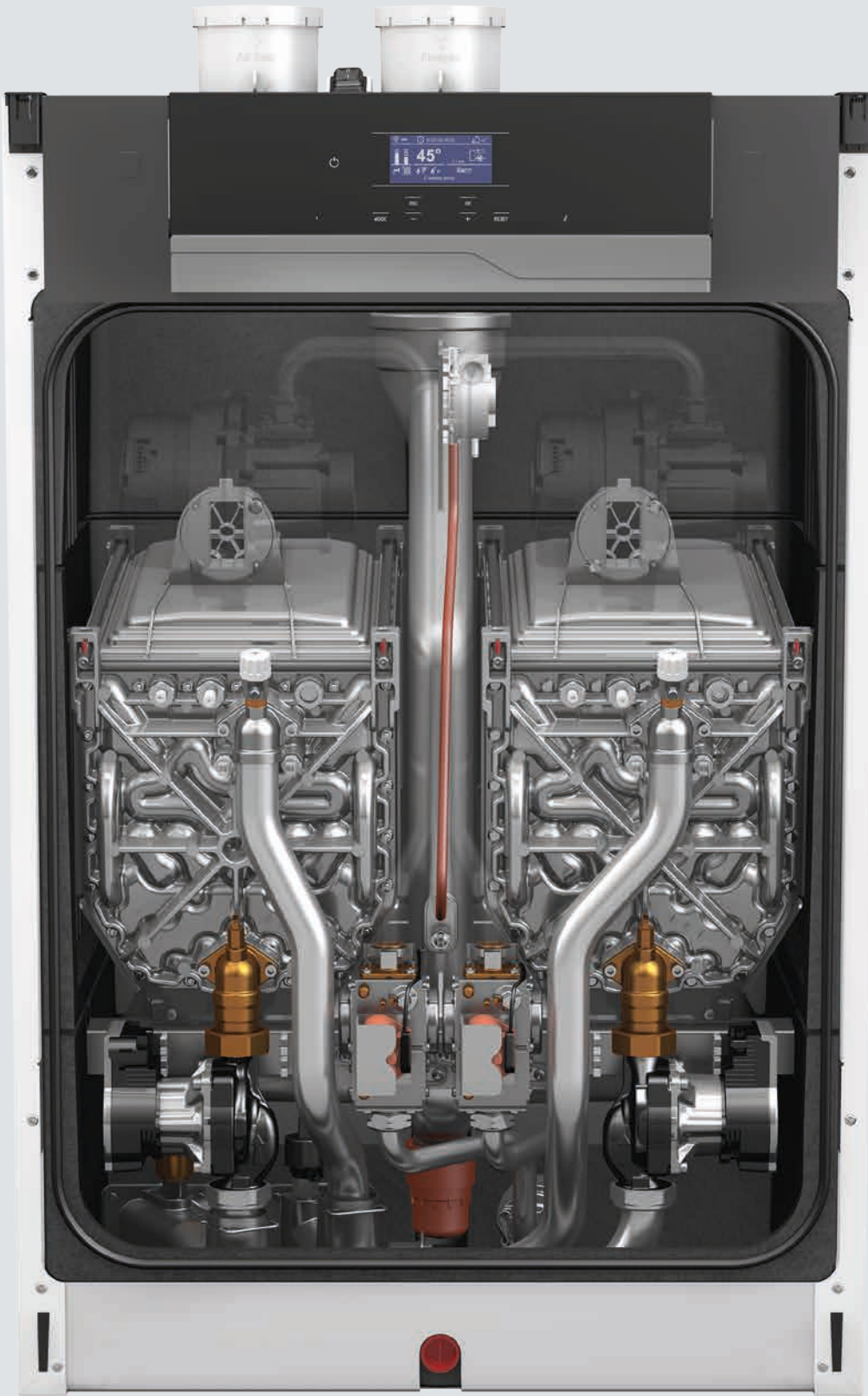
Dwa moduły grzewcze występują w kotłach o mocach powyżej 100 kW
